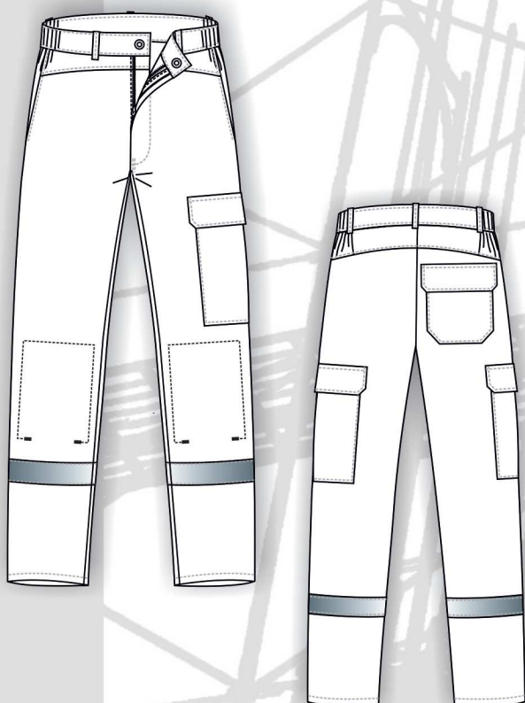
Poche mètre à rabat pression plastique cachée
